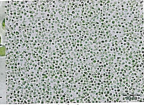
Diplosphaera chodatii
