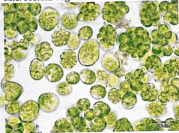
Myrmecia bisecta
