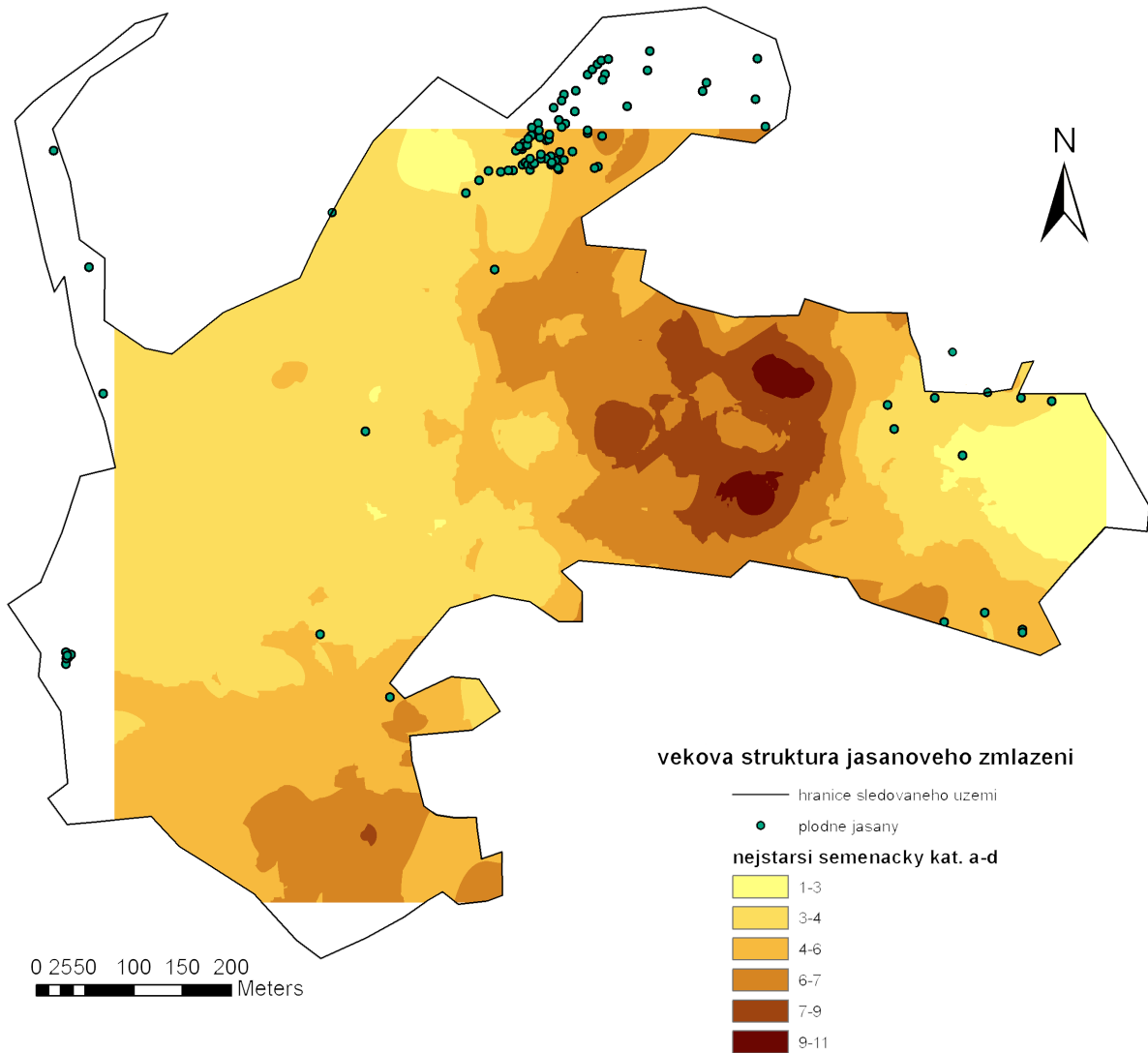
Obr. 15: Mapa věkové struktury (1-11 let) jasanových semenáčků kategorie a-d. Mapa byla vytvořena interpolací (metoda Kriging, ArcGIS 9 (ESRI 2005)) nejstaršího semenáčku v každém fytoecnologickém snímku.
