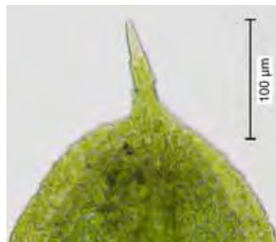
C. špička listu – var. aestiva
