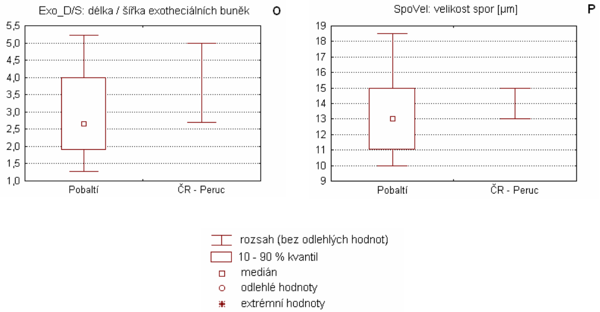
Obr. 1 O-P. Kvantitativní morfologické znaky sporofytu rostlin T. lingulata z Pobaltí a z ČR.
