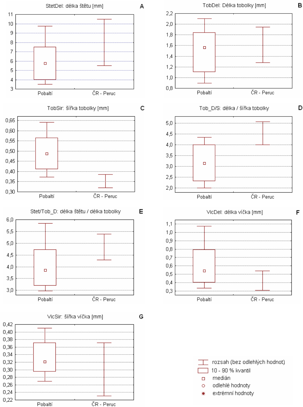
Obr. 1 A-G. Kvantitativní morfologické znaky sporofyту rostlin T. lingulata z Pobaltí a z ČR.
